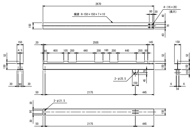
横 梁 詳 細 図 ＜S=1/20＞
