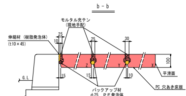
床版縦目地詳細図
