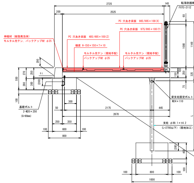
断 面 图 \langle S=1/20 \rangle
