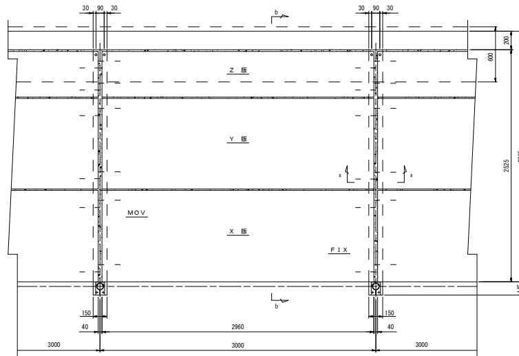
床版詳細図 ＜S=1/20＞
