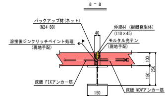
床版横目地詳細図
